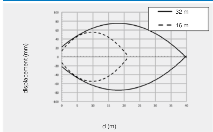
RXE/00-0* - RXR/00-0* parallel displacement
